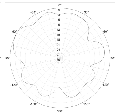
H-Plane Pattern
