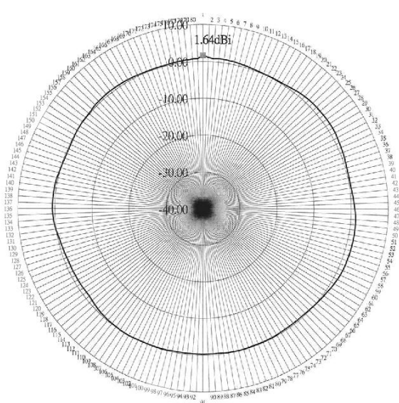
E-Plane
