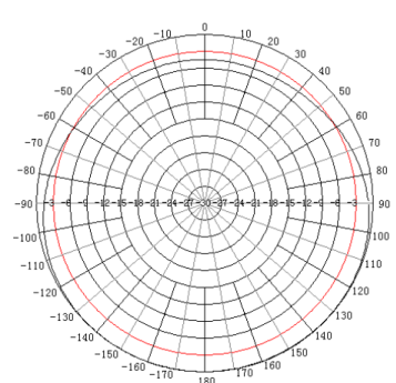
H-Plane Pattern
