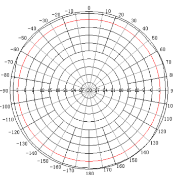
H-Plane Pattern
