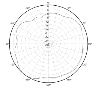
H-Plane Pattern
