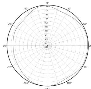
H-Plane Pattern
