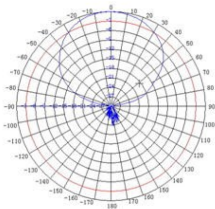
E-Plane
