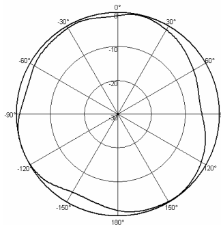
H-Plane Pattern
